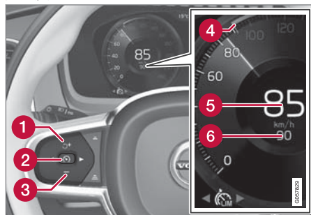
功能按鈕與符號 12 。
