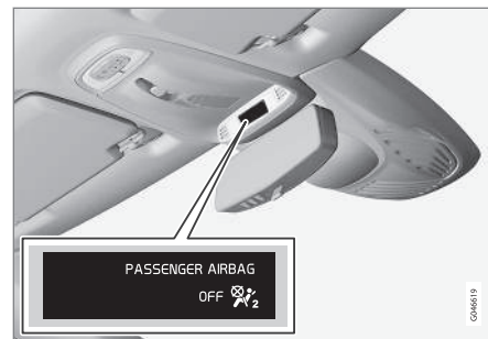
Indikering der viser, at passagerpladsens airbag er frakoblet.
