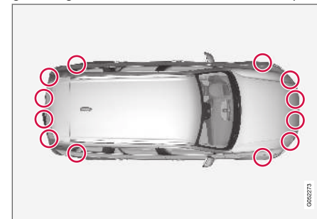
Parkeringssensorernas placering 132 .
