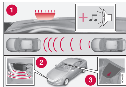
1. Lampka i dźwięk ostrzegawczy układu ostrzegającego o ryzyku kolizji 7 .
