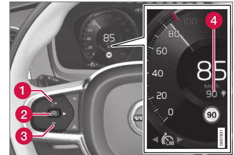
Funksjonenes knapper og symboler 25 .
