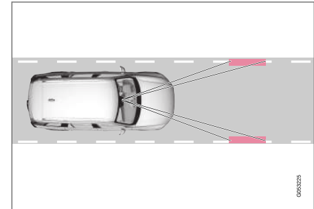
DAC låser bilens plassering i kjørefeltet.
