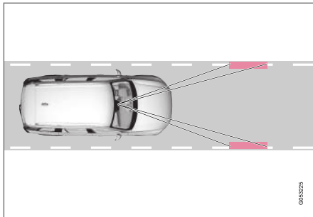
En kamera registrerer de malt kantlinjene i veien/filen.
