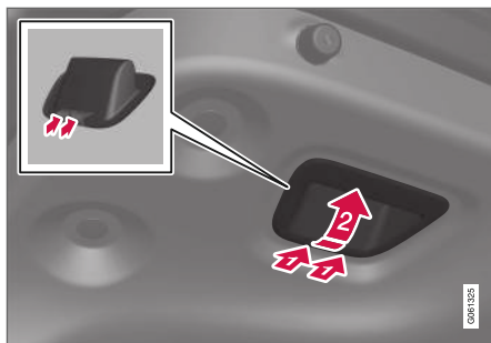
Uchwyt do zamykania pokrywy bagażnika.
