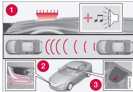
1. Akustisk och visuell varningssignal vid kollisionsrisk 22 .
