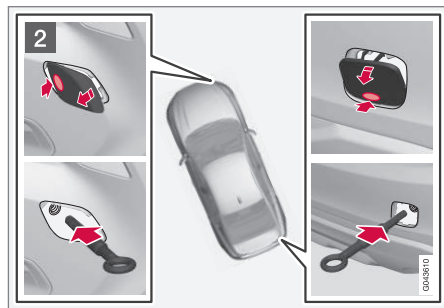
Remoção da tampa de cobertura à frente e atrás.
