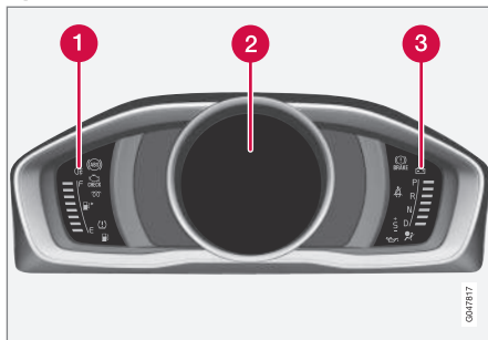
Spie di segnalazione e di allarme, strumentazione digitale.
