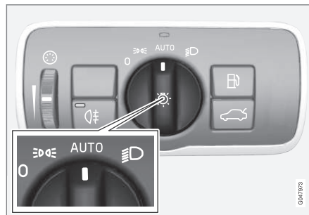
Disco selector do comando das luzes na posição AUTO .
