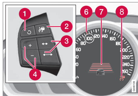
Controlo da velocidade adaptativo sem Limitador de velocidade 9 .
