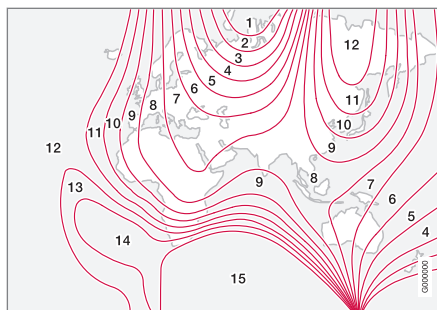
Zonas magnéticas.
