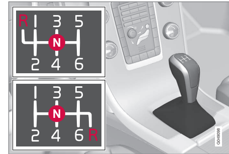
Schaltmuster 6-Gang-Getriebe.
