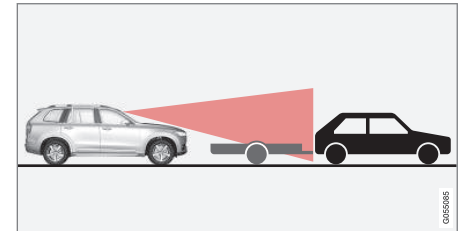
Lage aanhangwagen in radarschaduw.
