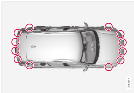
Localização dos sensores de estacionamento 109 .
