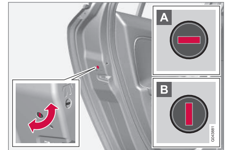
Portier handmatig vergrendelen. Niet te verwarren met het kinderslot (p. 191).
