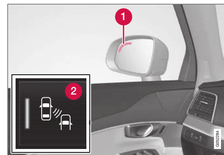
Ubicación del testigo de BLIS 72 .
