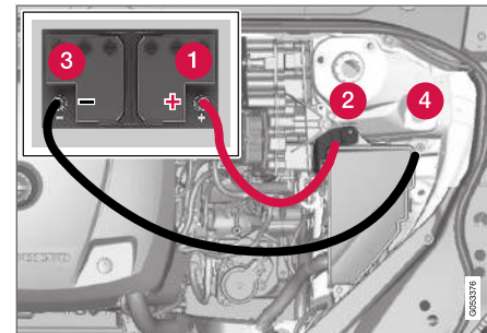
Ponto de carga para partida assistida do veículo.
