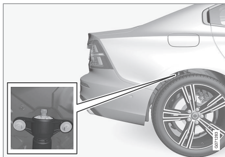
Localização do botão ajustador, roda traseira.
