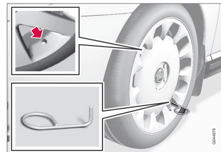
Instrumenti riteņu skrūvju plastmasas uzgaļu noņemšanai.
