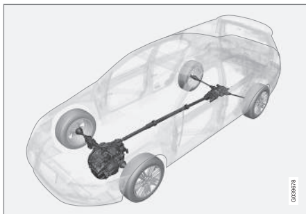
Princippet i firehjulstræk 7 .
