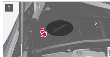
Expansionskär för kylsystem, vänsterstyrd bil.
