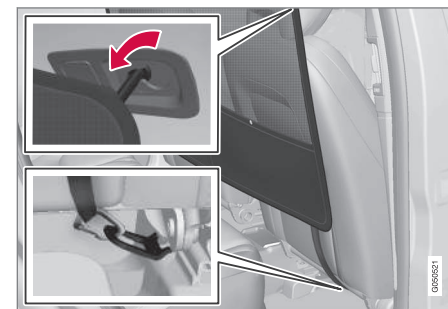
Montagem dianteira.
