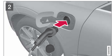
2 เปิดฝาปิดสำหรับการชาร์จ ถอดฝาปิดป้องกันของมือจับสำหรับการชาร์จออก แล้วกดมือจับเข้าไปในช่องเกิดสำหรับรถให้สุด
