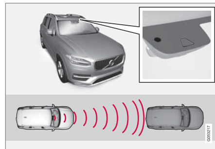
กล้องและชุดเรดาร์จะวัดระยะห่างจากรถคันหน้า
