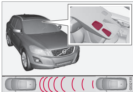
Finestre di trasmissione e ricezione del sensore laser 12 .
