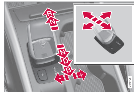
Panoramica della leva selettoria e delle posizioni del cambio.
