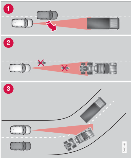
雷達單元的視野。 ❶ 有時雷達單元會太晚偵測到近距離的車輛，例如：行駛於您的車輛與前方車輛之間的車輛。
