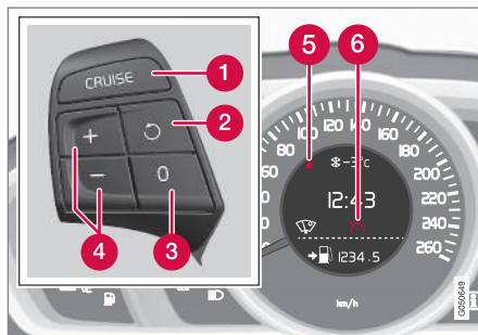
Teclado do volante e mostrador no automóvel sem Limiteador de velocidade 6 .
