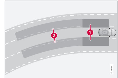
Princípio do BLIS: 1. Zona no ângulo morto. 2. Zona para veículo a aproximar-se rapidamente.
