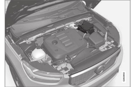
Käynnistysakku on sijoitettu moottoritilaan.
