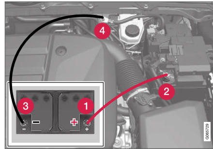
Käynnistyskaapelienn kiinnityspisteet.
