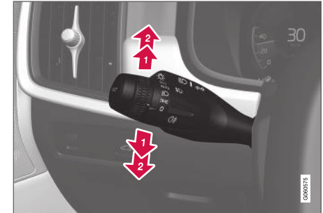
Suuntavalot.
