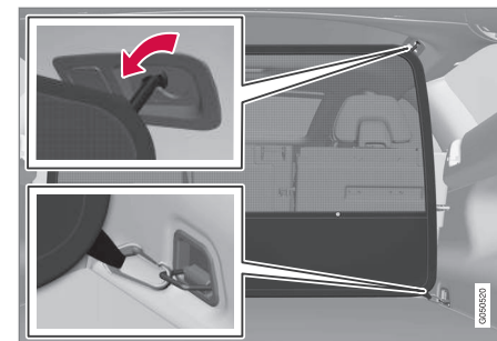
Montaggio posteriore.
