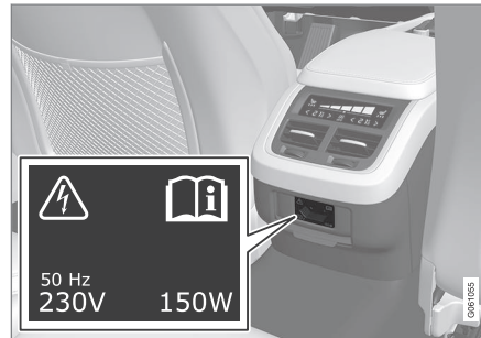
230-V-Steckdose in der Tunnelkonsole, Rücksitz.
