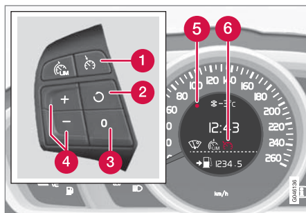
速度リミッター 2 装備の車両のステアリングリモコンとコンパインド・メーター・パネル
