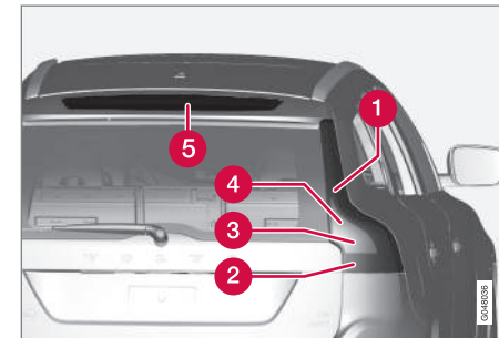
Lentille de feu arrière, côté droit
