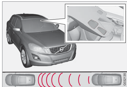
レーザーセンサーの送信/受信ウィンドウ 15
