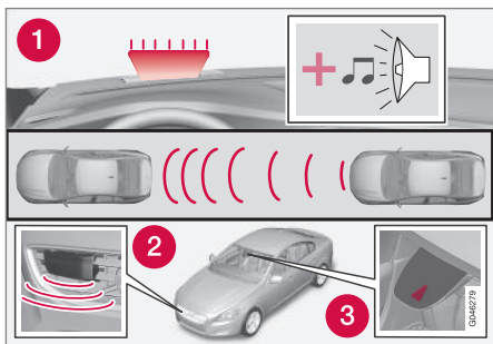
1. 碰撞警告系統警示燈及警示聲響 7 。
