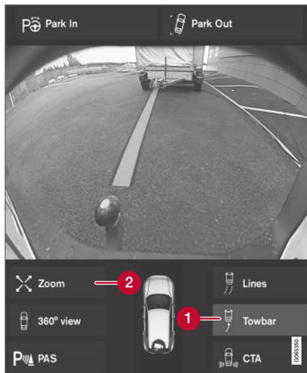
Gancio di traino e linea guida della traiettoria prevista 115 .
