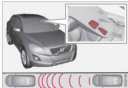
レーザーセンサーの送信/受信ウインド 13
