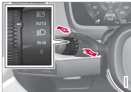
具有轉動環的方向盤撥桿開關。
