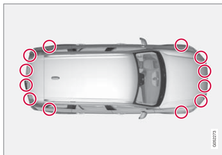
駐車感知器位置 138 。
