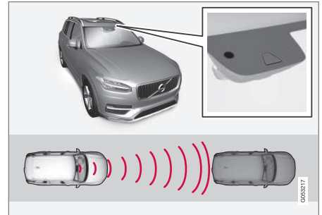
카메라 및 레이더 유닛은 앞차와의 간격을 측정합니다.
