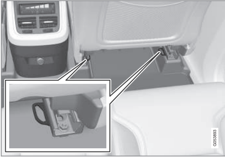
2열 좌석 앵커 위치.
