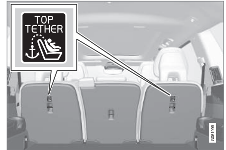
5인승 및 7인승: 고정 개소 위치는 등받이 뒤쪽에 심벌로 표시됩니다.
