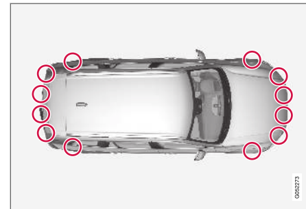
Parkeringssensorernas placering 124 .
