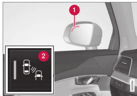
Localização das lâmpadas BLIS 72 .
