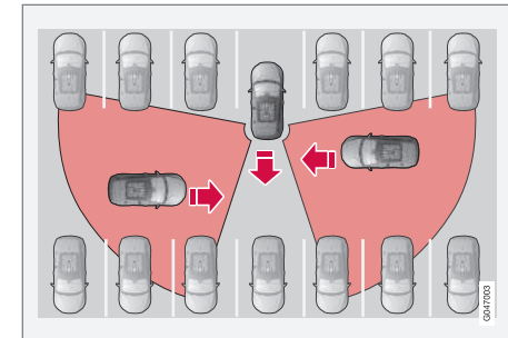
Principio del sistema CTA.
