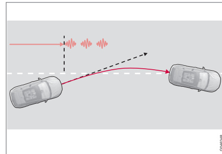
O LKA actua a direcção e avisa com vibrações no volante 26 .
