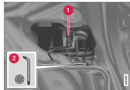
Lampunkotelo oikealla puolella peitekansineen.
