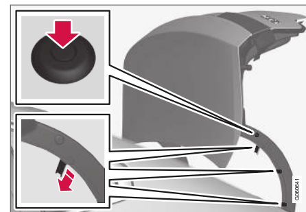
Saranan muovisuojuus on asennettu muoviniitillä ja kolmella jousilukolla.
