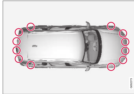
Pysäköintitunnistimien sijainti 137 .
