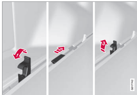
Arrimage de la charge avec les crochets d'arrimage mobiles .
