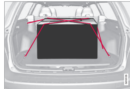
Charge arrimée aux points de fixation supérieurs et inférieurs.
