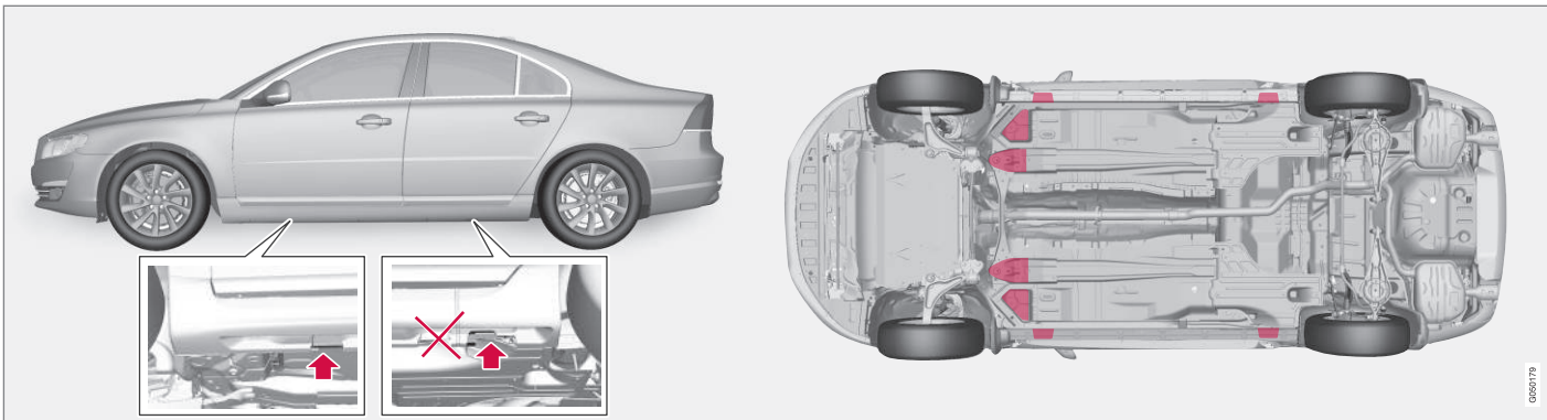
Punkty podpierania (strzałki) dla podnośnika dołączonego do samochodu i punkty podnoszenia (zaznaczone na czerwono).
