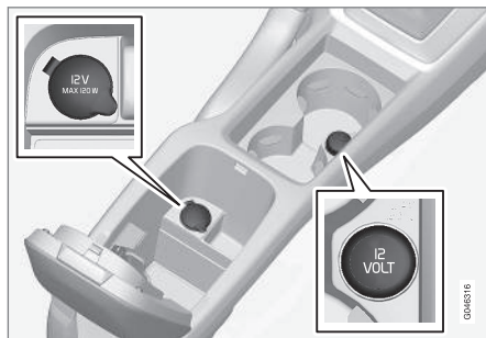
12 voltos aljzat az alagútkonzolban, első ülés.
