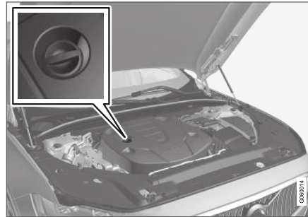
Påfyllingsrør 14 .
