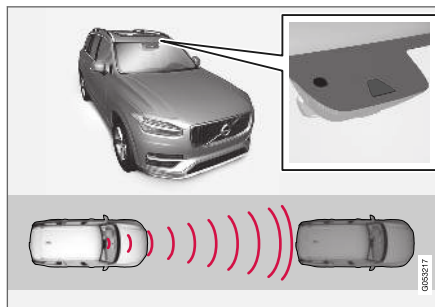
Kamera- og radarenheten måler avstanden til kjøretøyet foran 48 .
