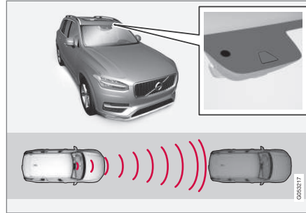
Kamera ve radar ünitesi öndeki araçla mesafeyi ölçer.
