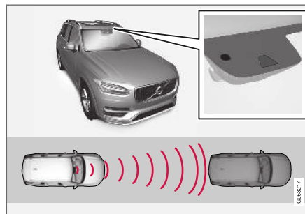
Kamera- och radarenhetens placering 70 .
