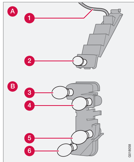
Polttimonpidin.
