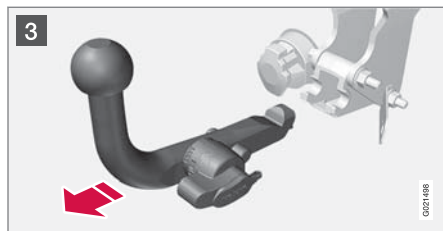
3 將鎖定輪一直向下轉動，直到停止位置。將拖車鉤向後及向上拉出時，將將鎖定輪固定在該位置。
